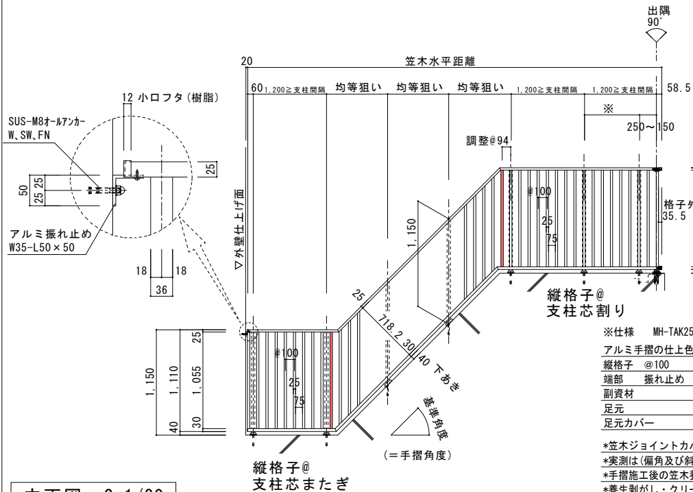
立面図 S=1/20
