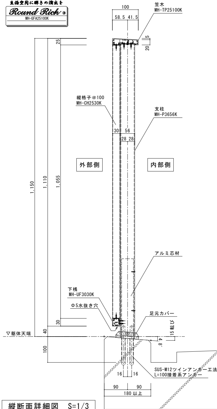
縦断面詳細図 S=1/3
