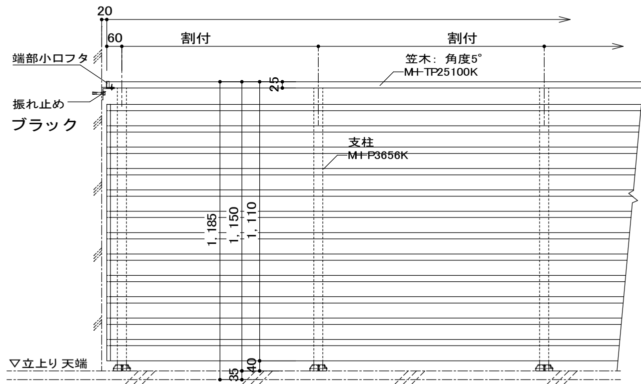
外観図
