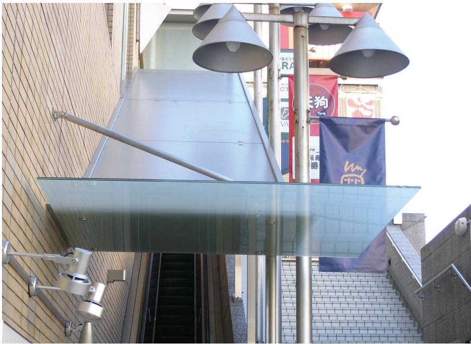
アルミ + ステンレス製 DPG 金具 強化合わせガラス製 世田谷区
