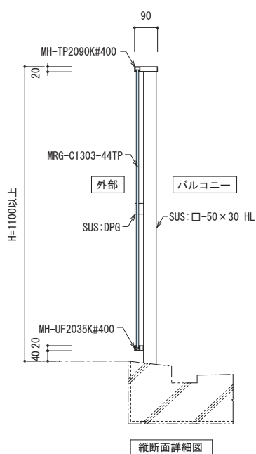
縦断面詳細図
